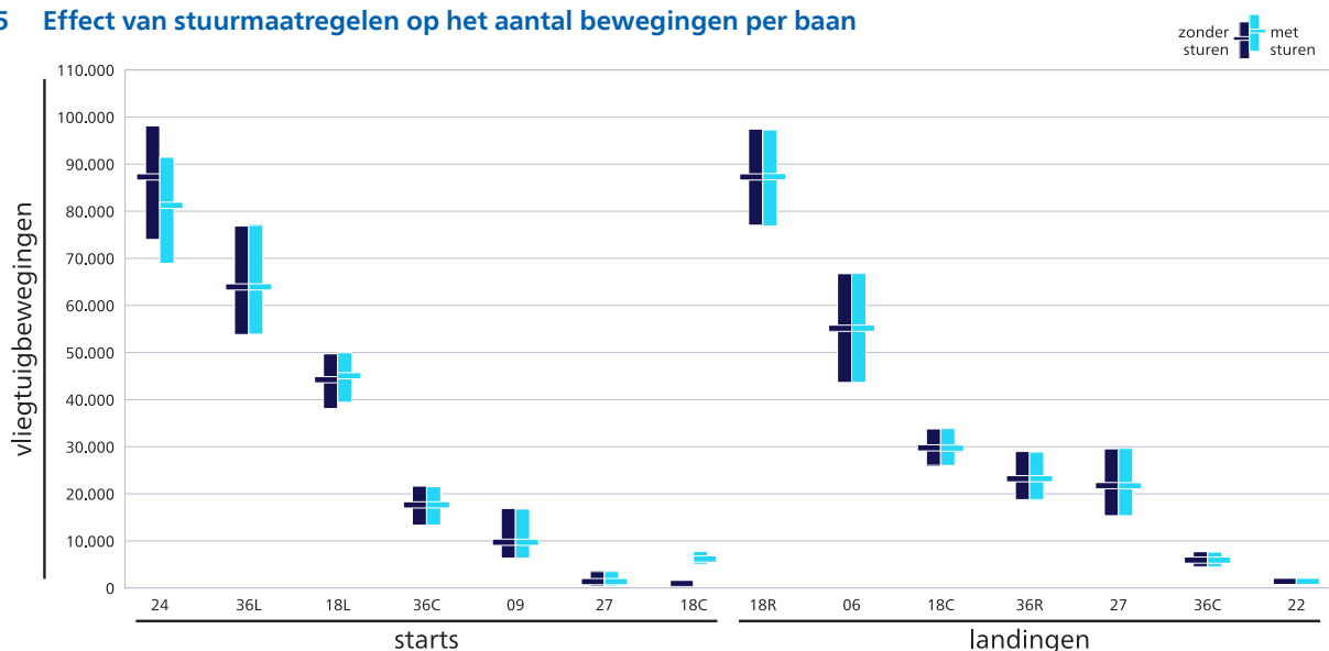
Figuur 7.5 Effect van stuurmaatregelen op het aantal bewegingen per baan
