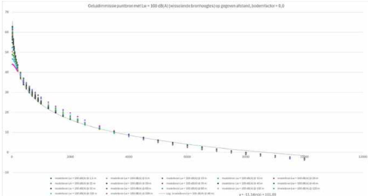
Figuur 5-3: Effect van een puntbron met een geluidvermogen L_{Wr} van 100 dB(A) op verschillende hoogtes van een geluidsbron
