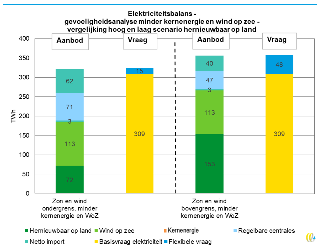
Figuur 9 – Elektriciteitsbalans, vergelijking ondergrensscenario en bovengrensscenario hernieuwbare opwek op land - gevoeligheidsanalyse minder kernenergie en windenergie op zee.
