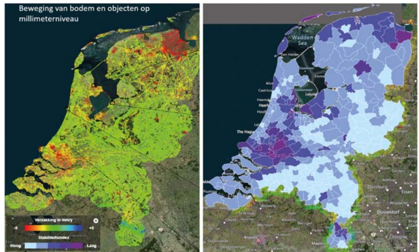
Figuur 9.3 Bodemdaling in Nederland
