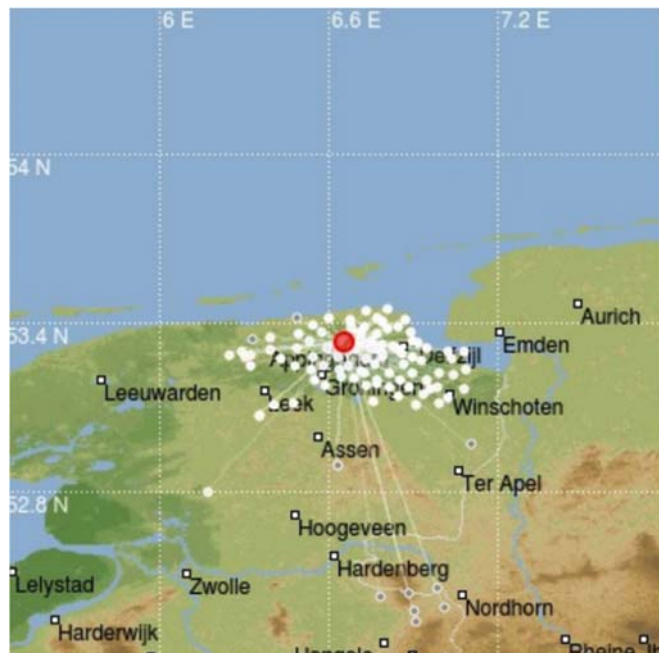
Figuur 9.1 Overzicht van de meetstations waar de beving van Westervijtwerd op 22 mei 2019 is geregistreerd
