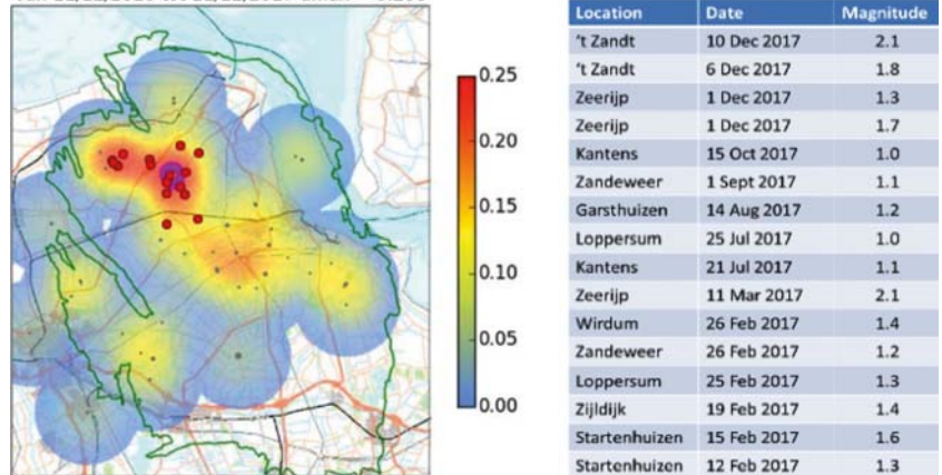
Figuur 7.1 Analyse van de overschrijding van het aantal aardbevingen groter dan magnitude 1 per vierkante kilometer in 2017
