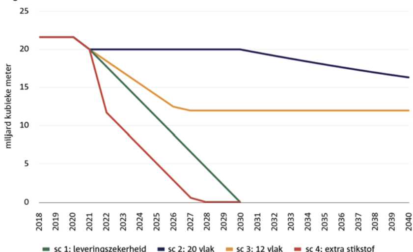
Figuur 7.4 Afbouwscenario's
