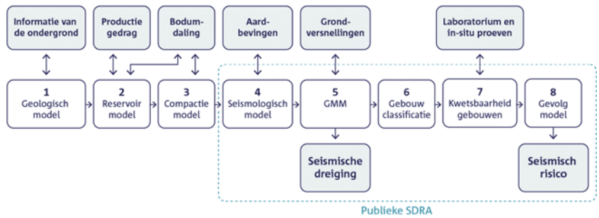
Figuur 9.2 Schematisch overzicht van de rekenmodellen die nodig zijn om de risico's van de gaswinning te berekenen in de seismische risicoanalyse
